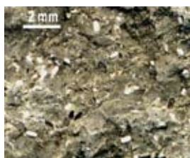
Nagromadzenie skorupki małżoraczek na powierzchni ilowca.
