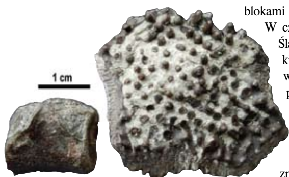
Krąg i tarczka kostna drobnego labiryntodonta Plagiosaurus .
