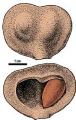
Rekonstrukcja luszki nasiennej z Lipia Śląskiego w widoku od dołu i z góry (nie ma listka okrywowego, jak u Stachyotaxus ), z przedstawionym tylko jednym nasionem w zagłębieniu częściowo osłoniętym epimatium.
